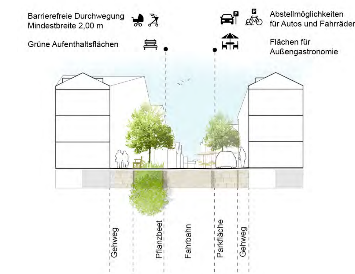
Vitusstraße, Schnitt M 1 : 200
